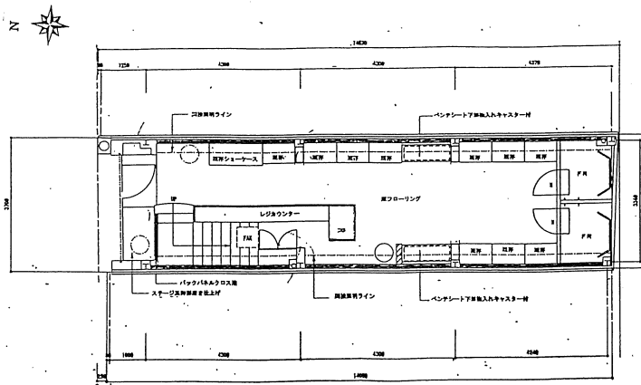
1階 平面図
