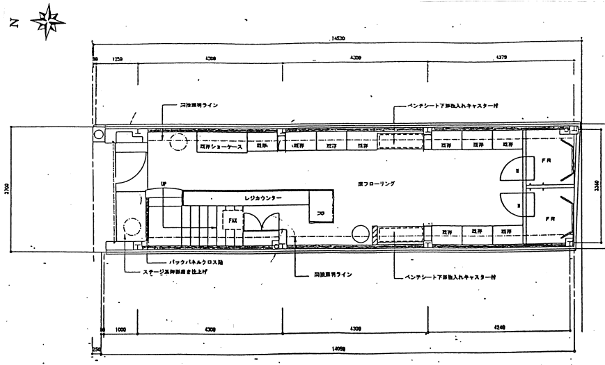
1階 平面図
