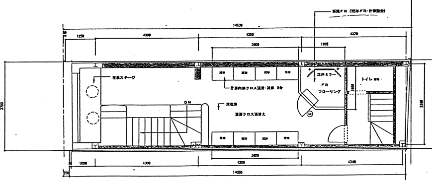
2階 平面図
