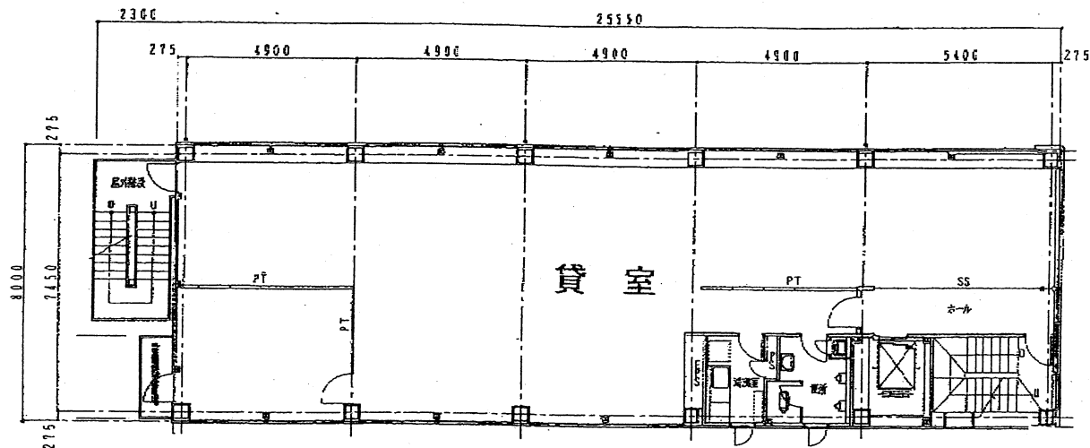
4階 平面図
